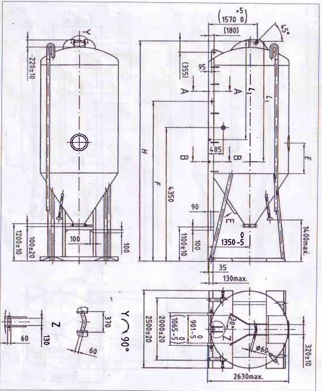
Bild 3: Anschlussmaße gemäß DIN 30734
