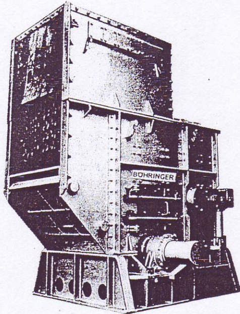
Abb. 19: Prallbrecher PB
