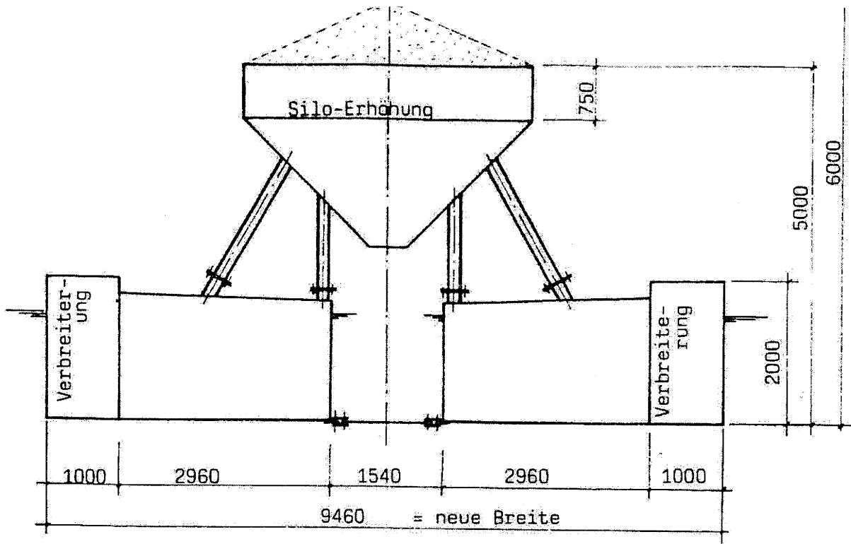
Mittschiffs - Querschnitt
