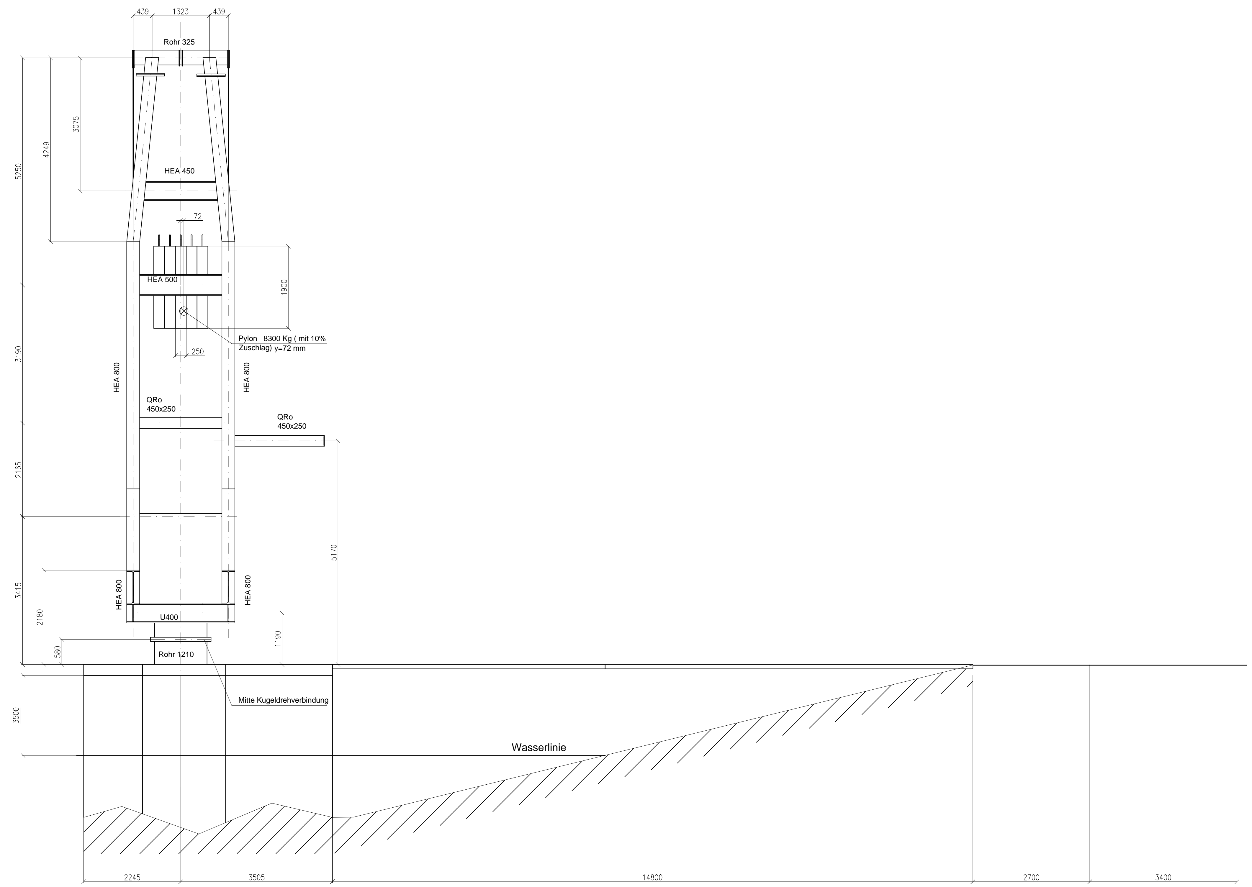
Schnitt A - A (ohne Ausleger)
