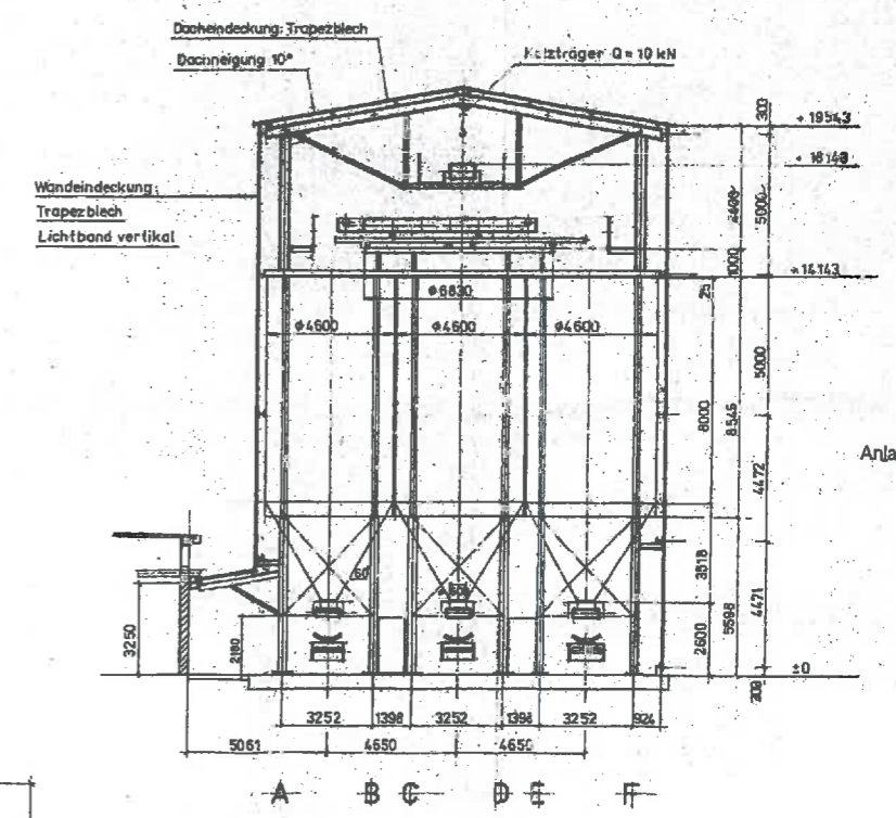
Schnitt A-B
