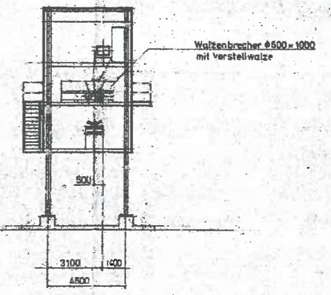
Schnitt A-B
