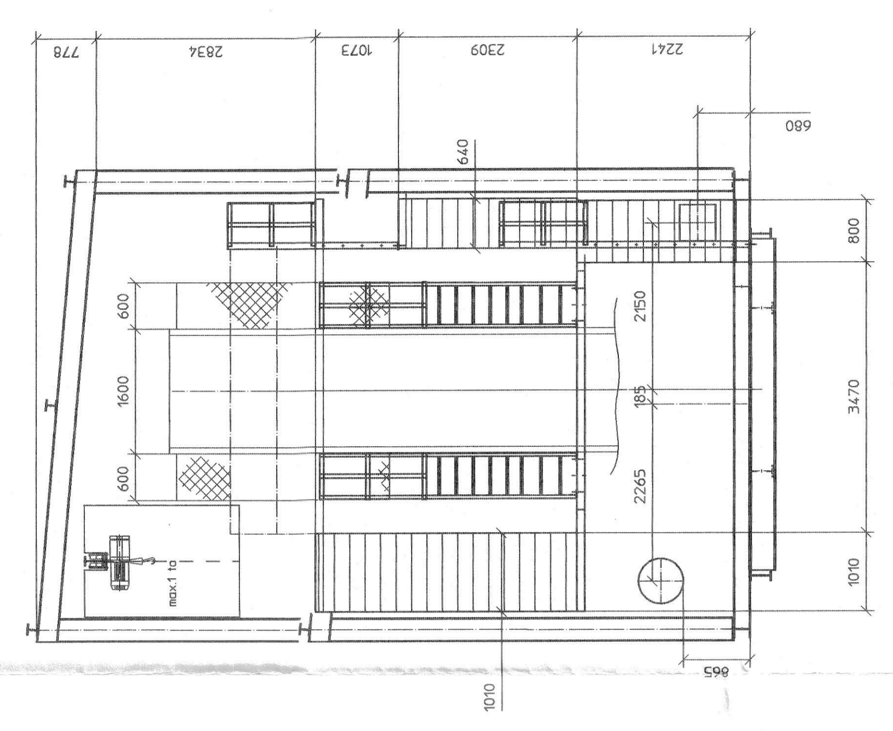
Ansicht A-A
