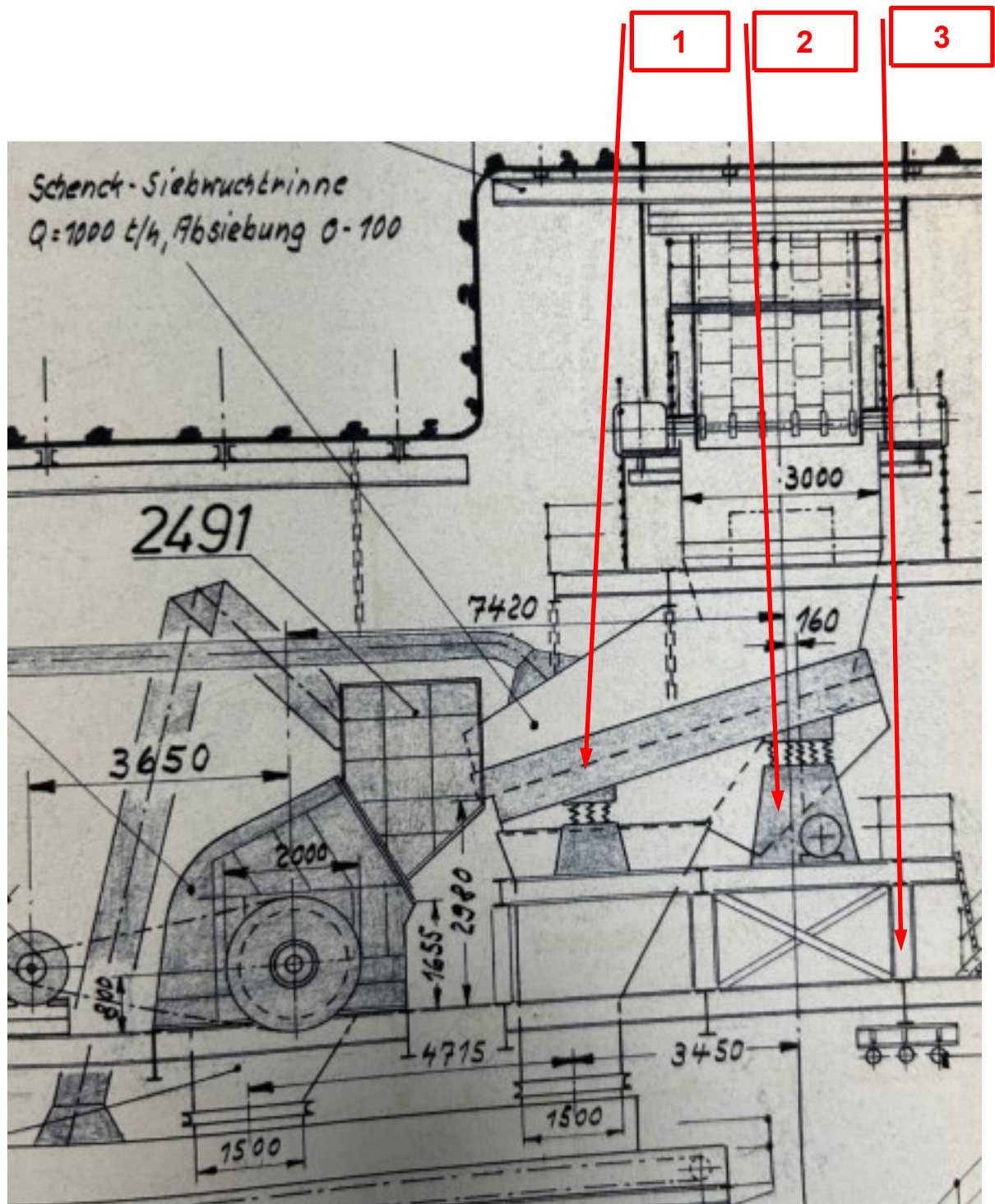
Abb. 1: Die Position dieser Maschine im Kalibergwerk (Ein Ausschnitt aus einer technischen Zeichnung)
