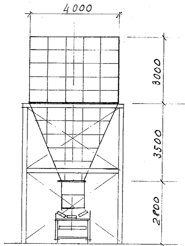
ANSICHT B-B
