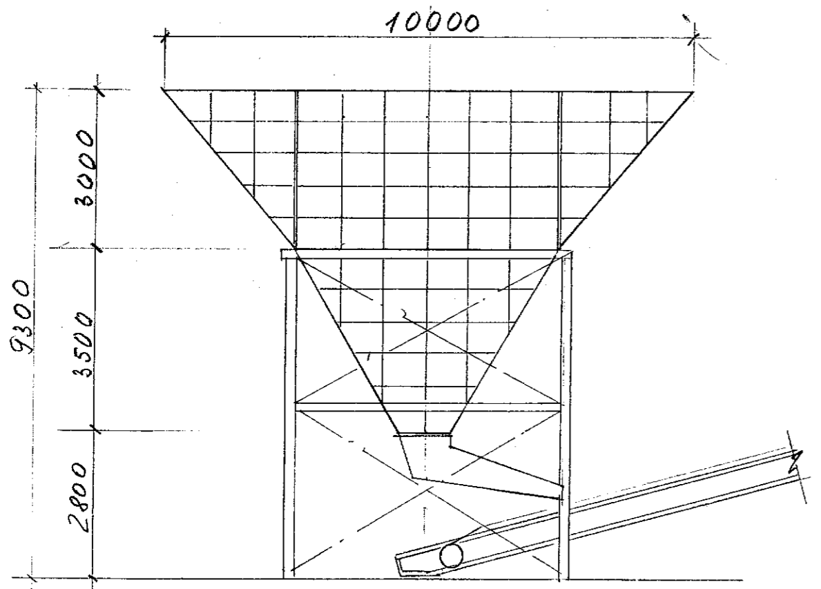
ANSICHT A-A
